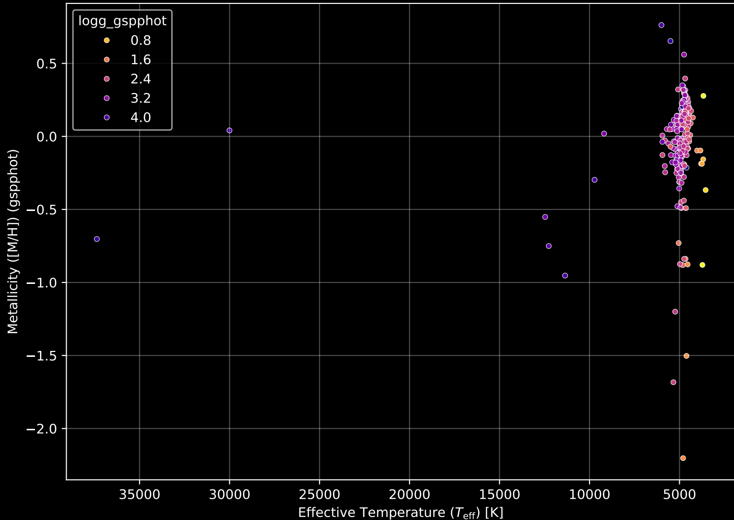
APOGEE DR17 Field: [049+06] Stellar Population Parameters (n= 293)
